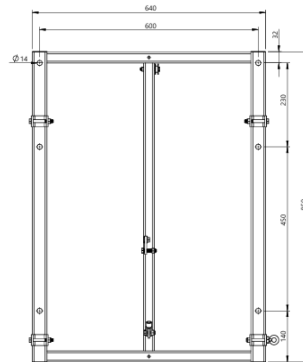
Seinärunko scale 1:7
